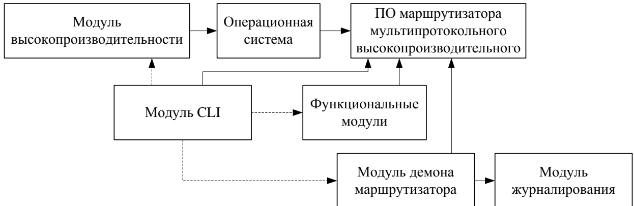
Рисунок 1 - Структурная схема программы
